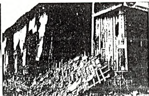
Foto 26. Santiago de Maria. Efectos del terremoto en una construcción de bahareque.
