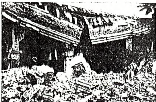
Foto 6. Chinameca. La destrucción del techo de bóveda del templo; se reconoce la ligera armazón de acero.
