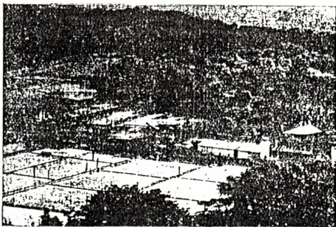
Foto 7. Beneficio «San José». Vista al suroeste; se reconoce la chimenea doblada hacia el oriente.
