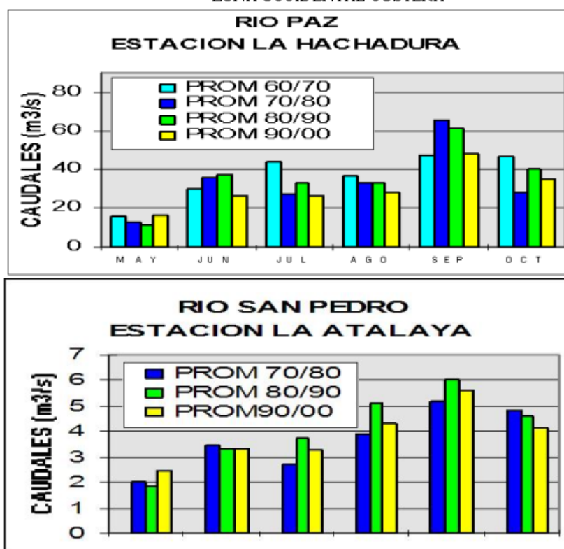
FIGURA 1.21. PROMEDIOS DECADEALES DE CAUDAL EN EPOCA LLUVIOSA ZONA OCCIDENTAL COSTERA
