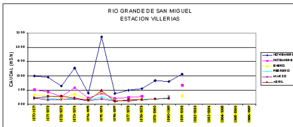
FIGURA 1.6. CAUDALES PROMEDIOS HISTORICOS EN LOS MESES DE NOVIEMBRE A ABRIL CUENCA RIO GRANDE DE SAN MIGUEL
