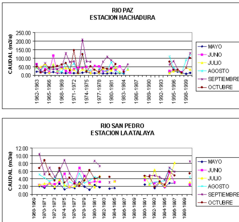
FIGURA 1.18. CAUDALES PROMEDIOS HISTORICOS EN LA EPOCA LLUVIOSA ZONA OCCIDENTAL COSTERA
