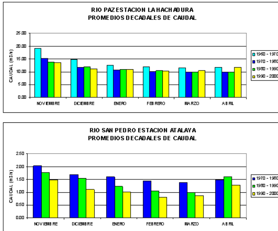
FIGURA 1.3. PROMEDIOS DECADALES DE CAUDAL EN EPOCA SECA ZONA OCCIDENTAL COSTERA
