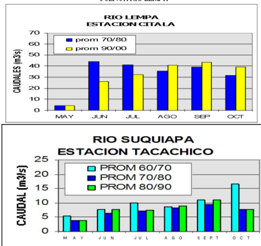
FIGURA 1.22. PROMEDIOS DECADEALES DE CAUDAL EN EPOCA LLUVIOSA CUENCA RIO LEMPA
