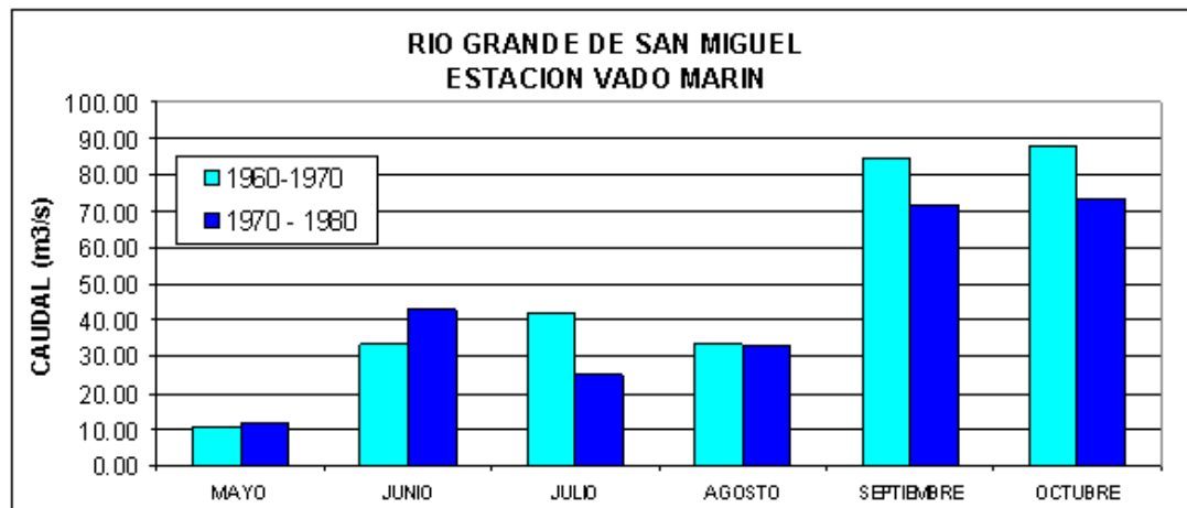
FIGURA 1.23. PROMEDIOS DECADALES DE CAUDAL EN EPOCA LLUVIOSA CUENCA RIO GRANDE DE SAN MIGUEL
