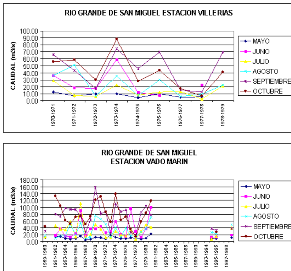
FIGURA 1.20. CAUDALES PROMEDIOS HISTORICOS EN LA EPOCA LLUVIOSA CUENCA RIO GRANDE DE SAN MIGUEL
