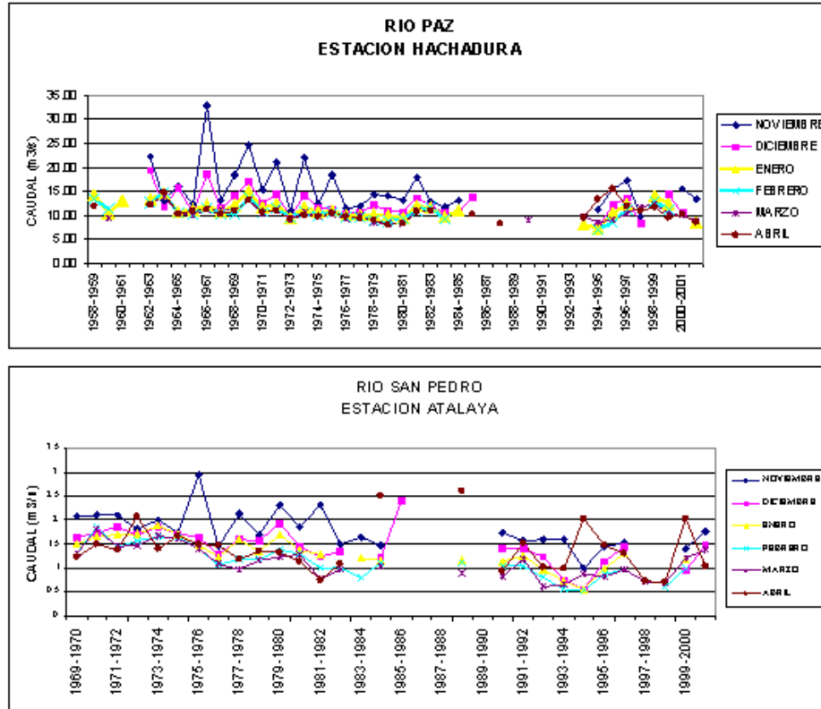
FIGURA 1.2. CAUDALES PROMEDIOS HISTORICOS EN LOS MESES DE NOVIEMBRE A ABRIL ZONA OCCIDENTAL COSTERA
