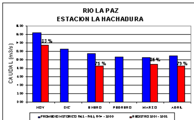
FIGURA 1.8. ANALISIS ESTACIONAL EN EL PERIODO NOVIEMBRE 2001-ABRIL 2002 ZONA OCCIDENTAL COSTERA
