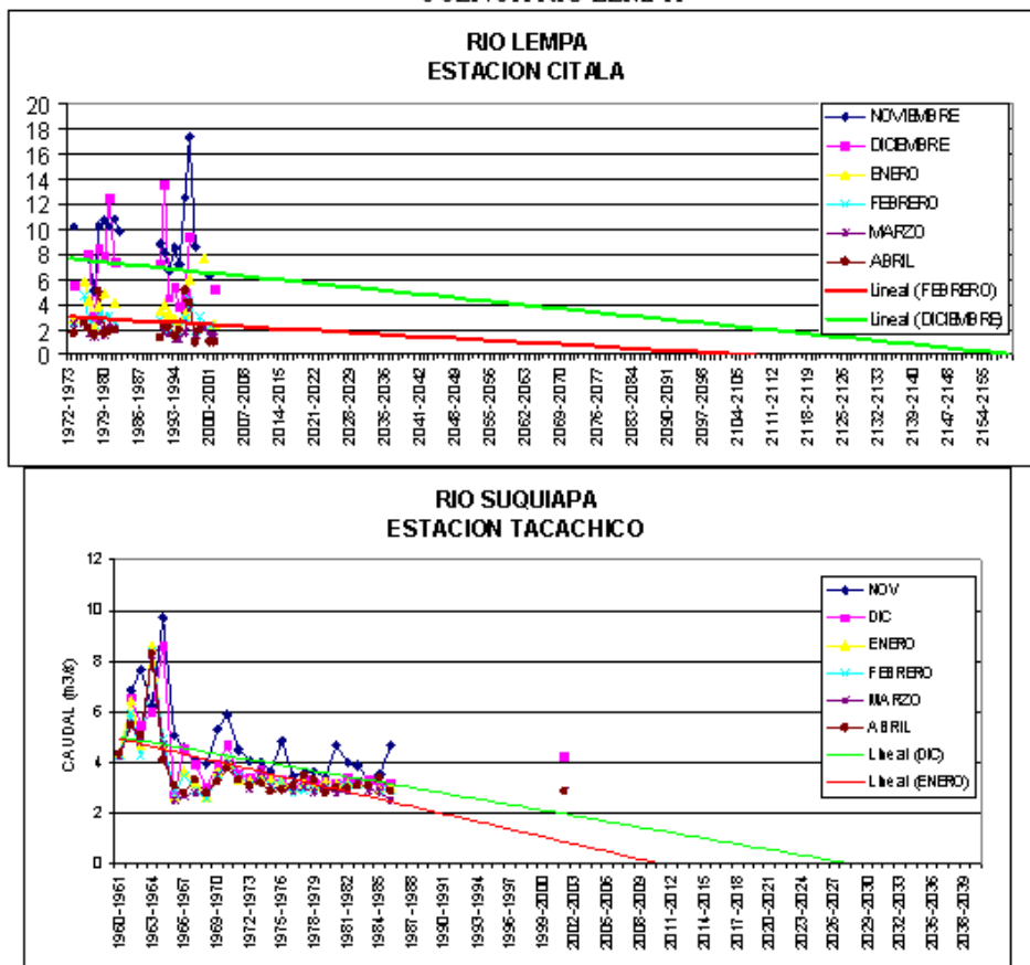
FIGURA 1.16. LINEAS DE TENDENCIA DE CAUDALES CUENCA RIO LEMPA
