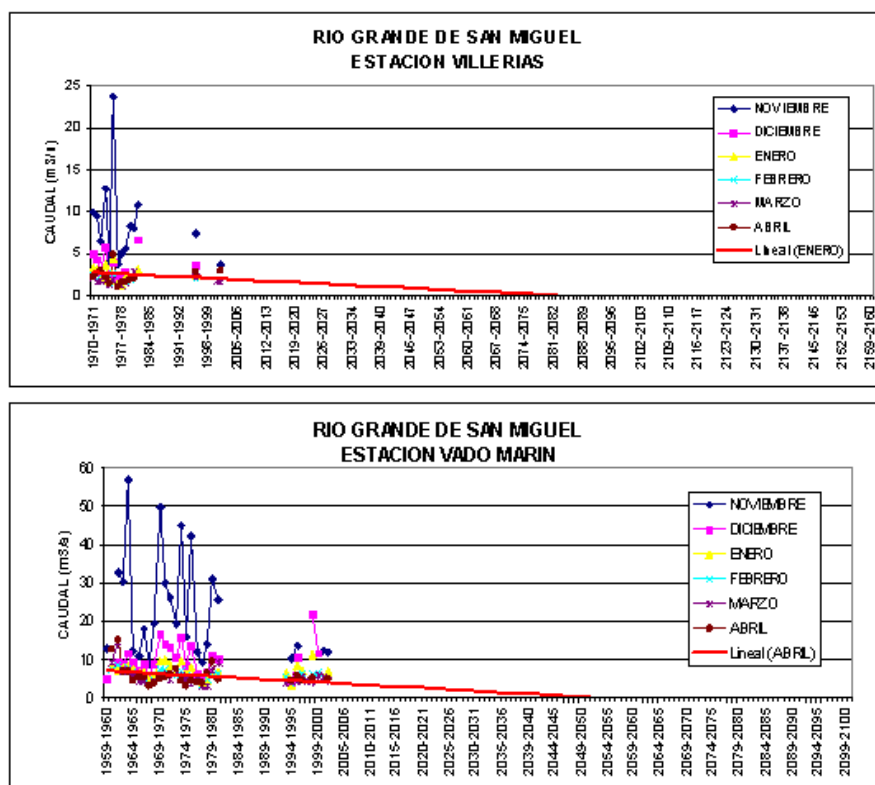
FIGURA 1.17. LINEAS DE TENDENCIA DE CAUDALES CUENCA RIO GRANDE DE SAN MIGUEL
