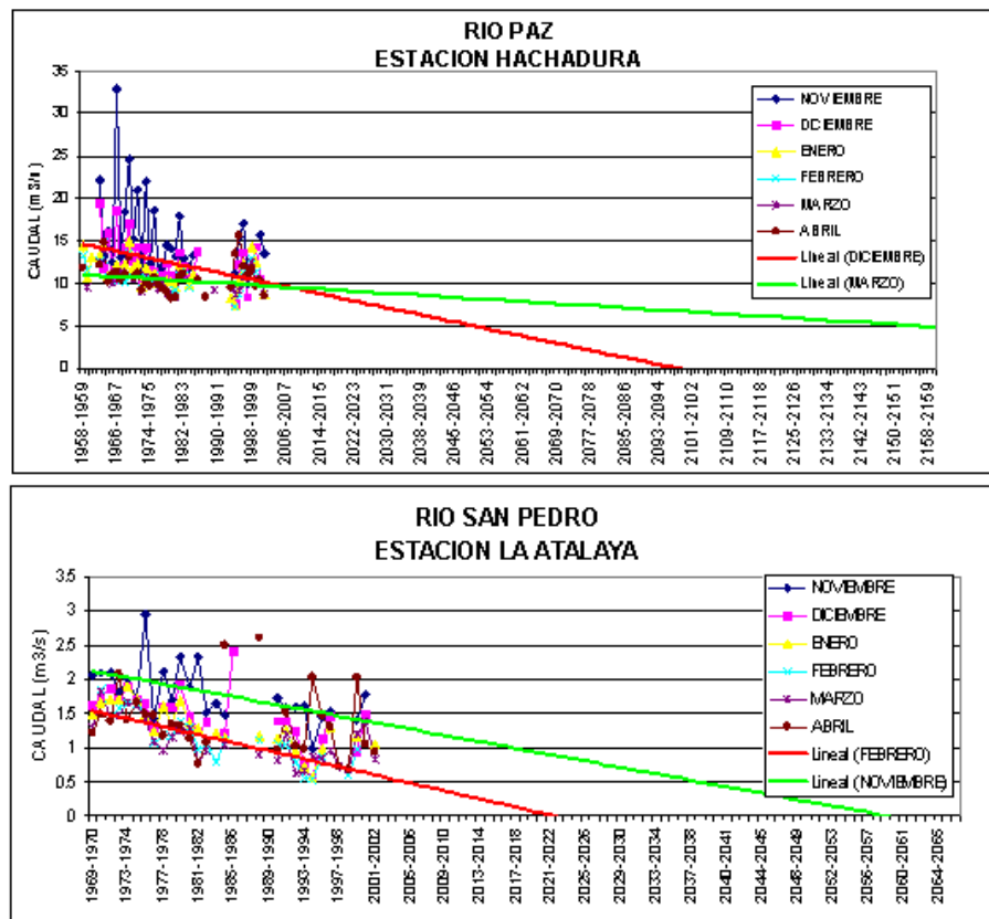
FIGURA 1.15. LINEAS DE TENDENCIA DE CAUDALES ZONA OCCIDENTAL COSTERA
