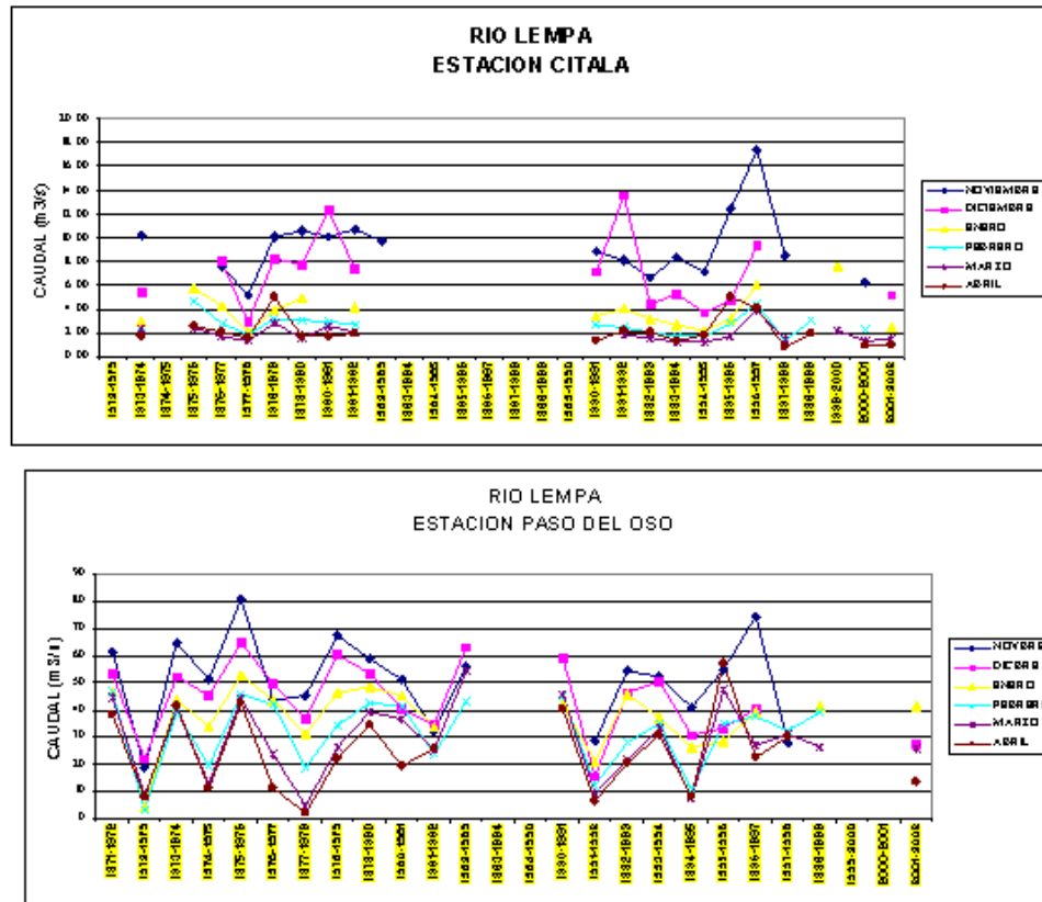
FIGURA 1.4. CAUDALES PROMEDIOS HISTORICOS EN LOS MESES DE NOVIEMBRE A ABRIL CUENCA RIO LEMPA
