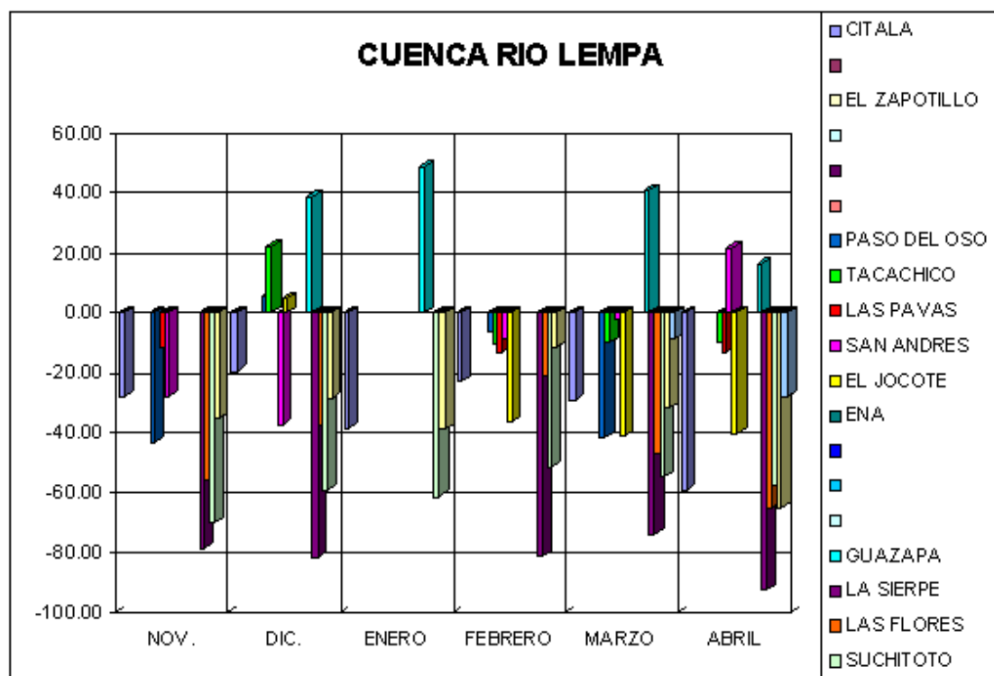
FIGURA 1.12. DIFERENCIAS PORCENTUALES DEL PERIODO NOVIEMBRE 2001 - ABRIL 2002 RESPECTO A LA DECADA 1970 - 1980
