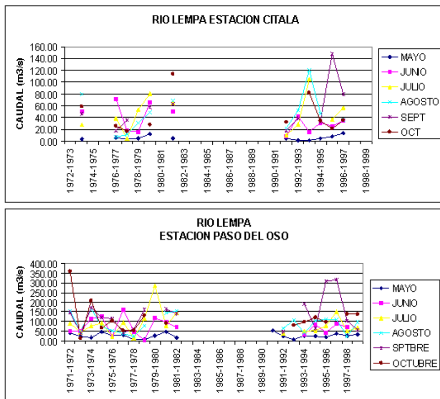
FIGURA 1.19. CAUDALES PROMEDIOS HISTORICOS EN LA EPOCA LLUVIOSA CUENCA RIO LEMPA
