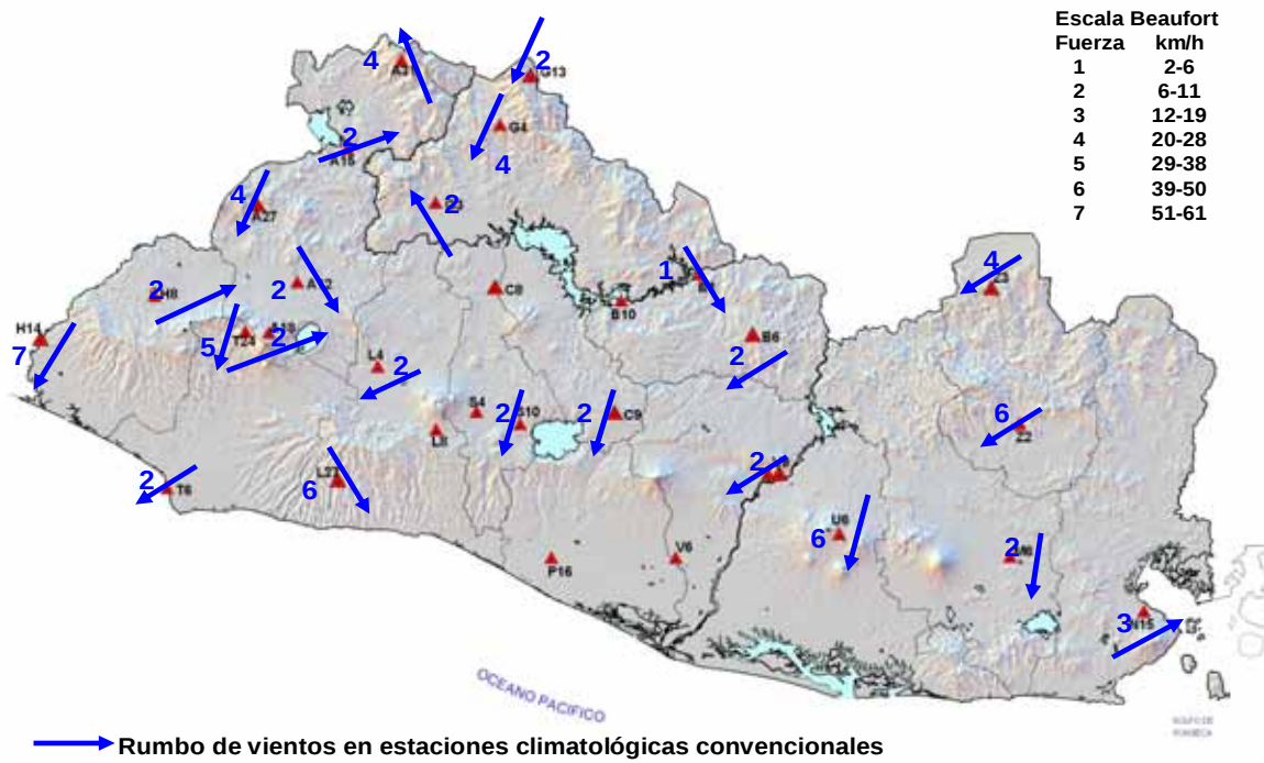
Mapa No 3: Rumbo y fuerza del viento en escala Beaufort, para el día 19 de mayo durante el temporal Adrian
