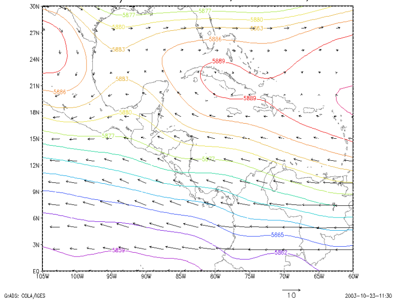
Promedio GPM/Vientos Mes Junio, 1982-1994, 500HPa
