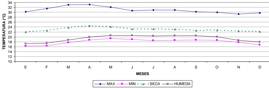
FIGURA 11 : TEMPERATURAS SECA, HUMEDA Y EXTREMAS EN SOYAPANGO
