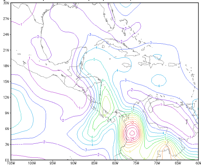
Rango de Precipitacion Total(mm/diarios), Mes Enero, 1982-1994
