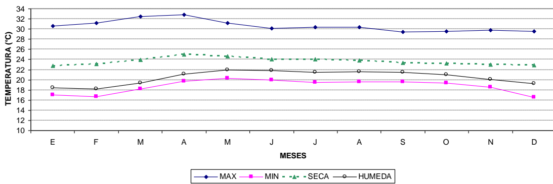
FIGURA 12 : TEMPERATURAS SECA, HUMEDA Y EXTREMAS EN ILOPANGO
