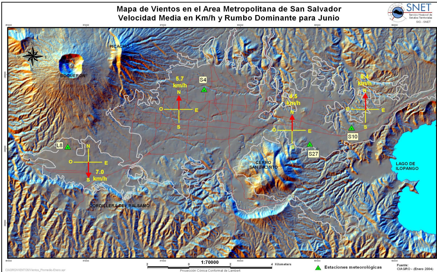
Mapa 11: Mapa vientos en estaciones meteorológicas, mes de Junio, AMSS.
